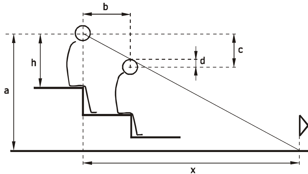
Рис. 14 Линия видимости для зрителей
