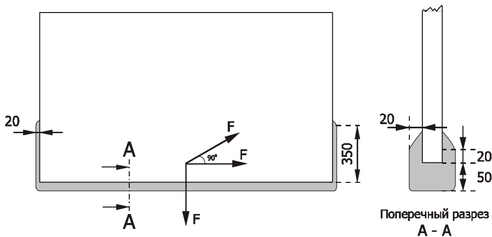
Рис. 7 Обивка щита
